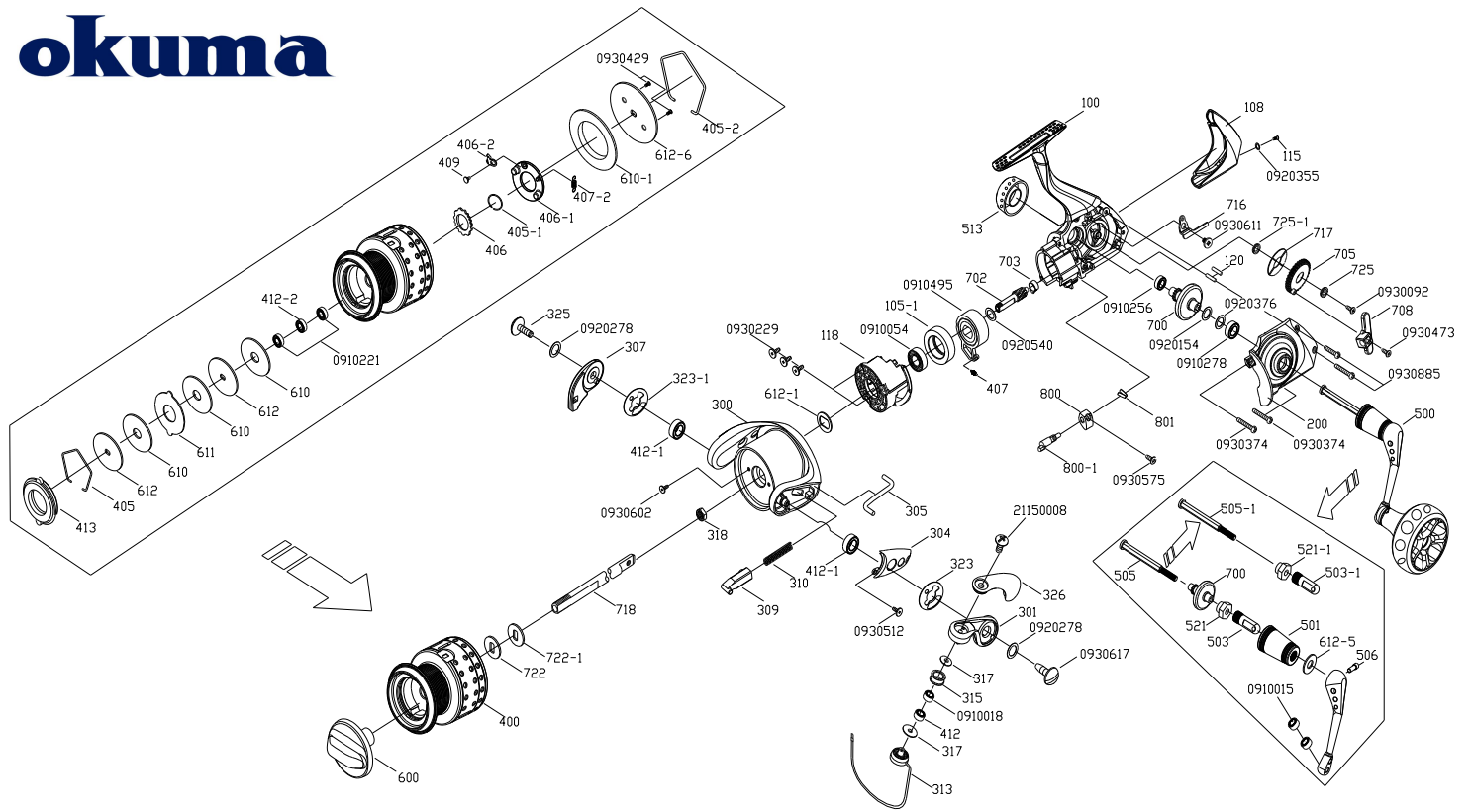
SA II-3000 零件清單
