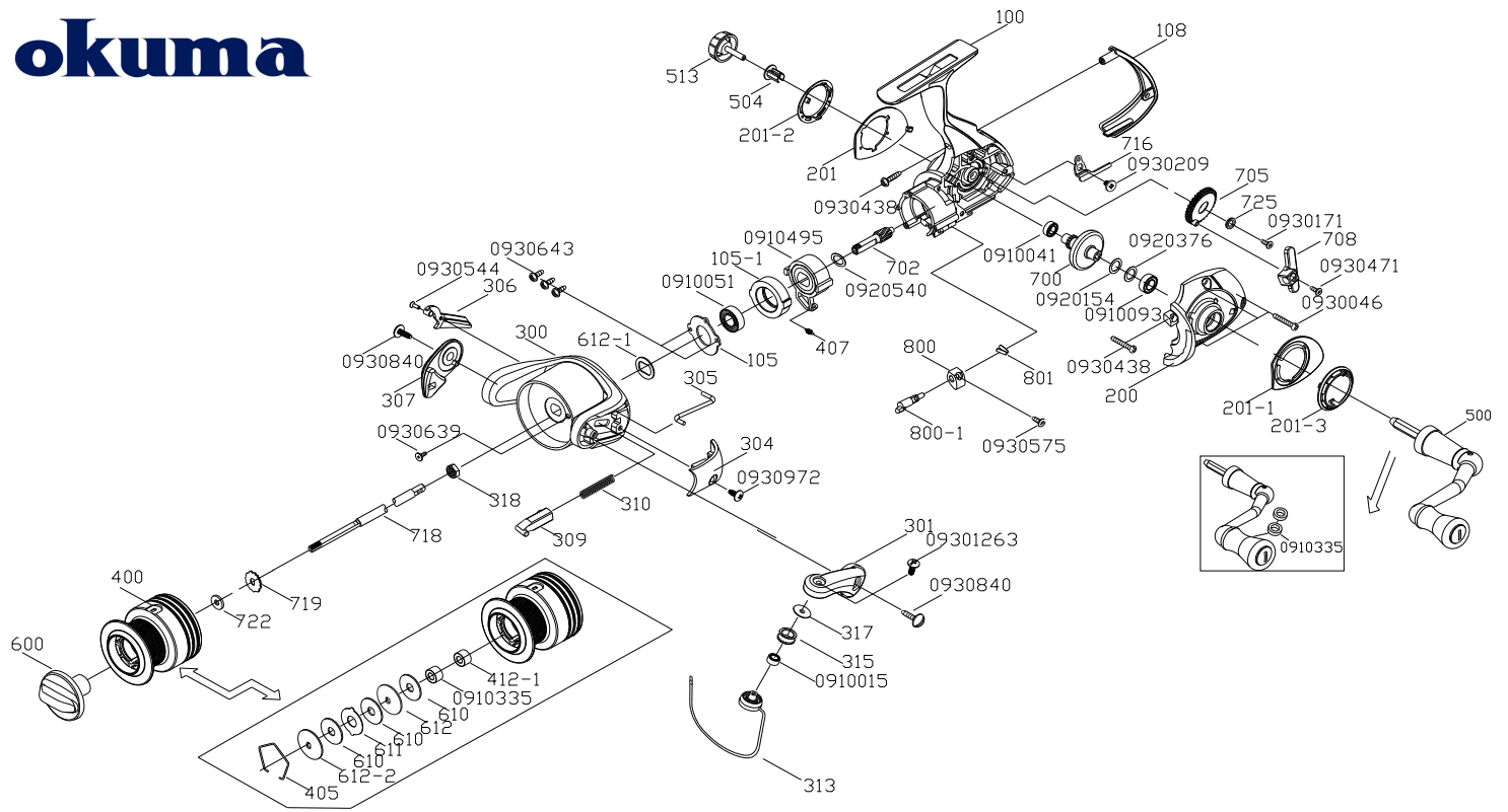
Pisces II-4000 零件清單
