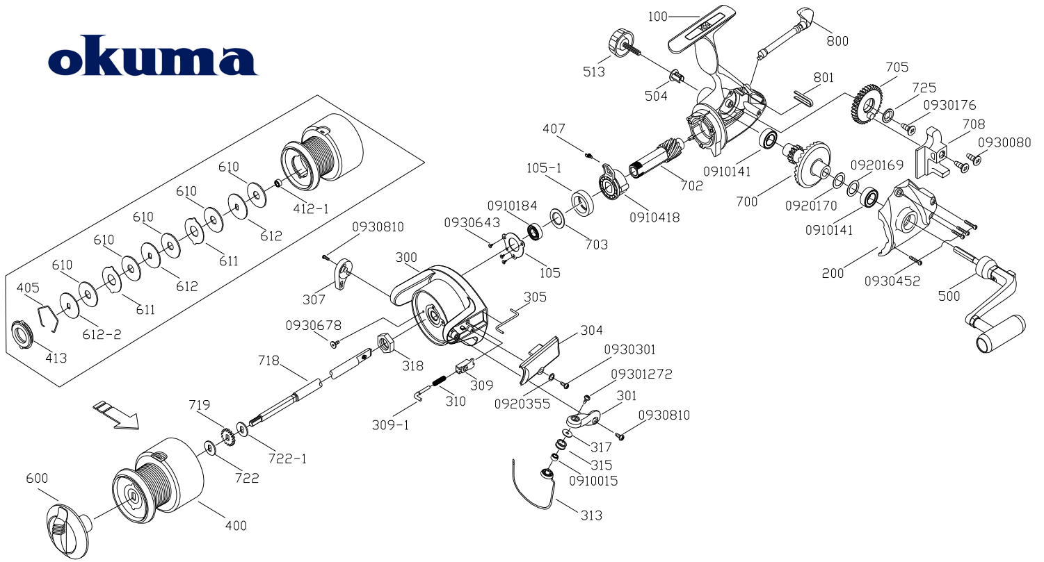
ANNEXER-6000 零件清單
