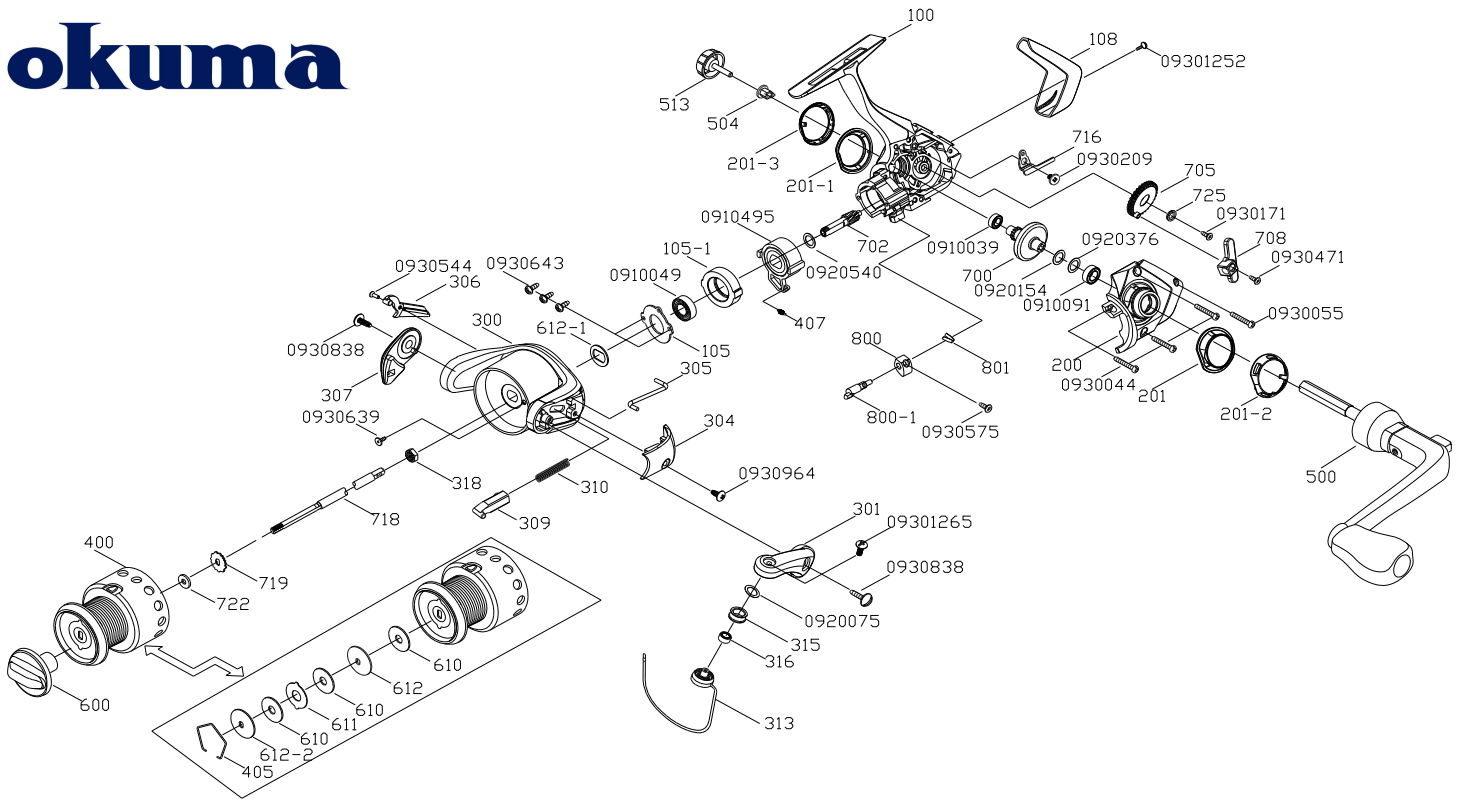
SPa-3000 零件清單
