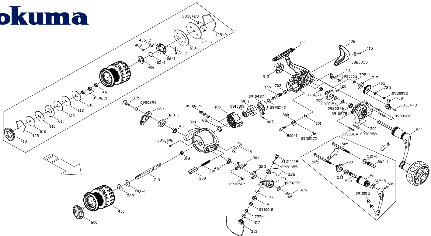
SA II-5000 零件清單
