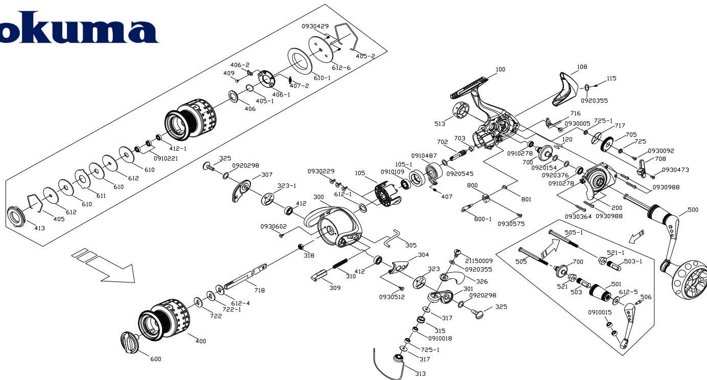
SA II-8000S 零件清單
