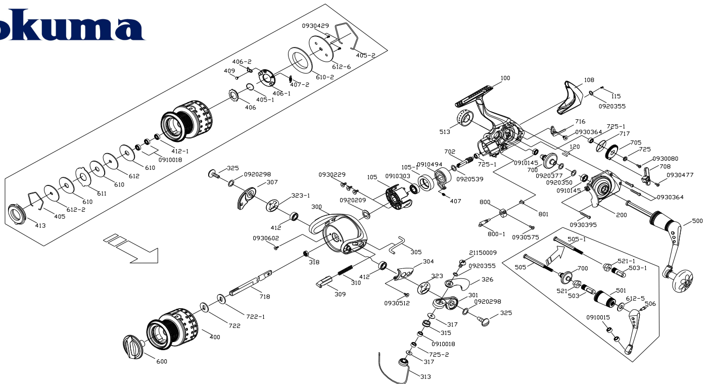
SA II-10000 零件清單
