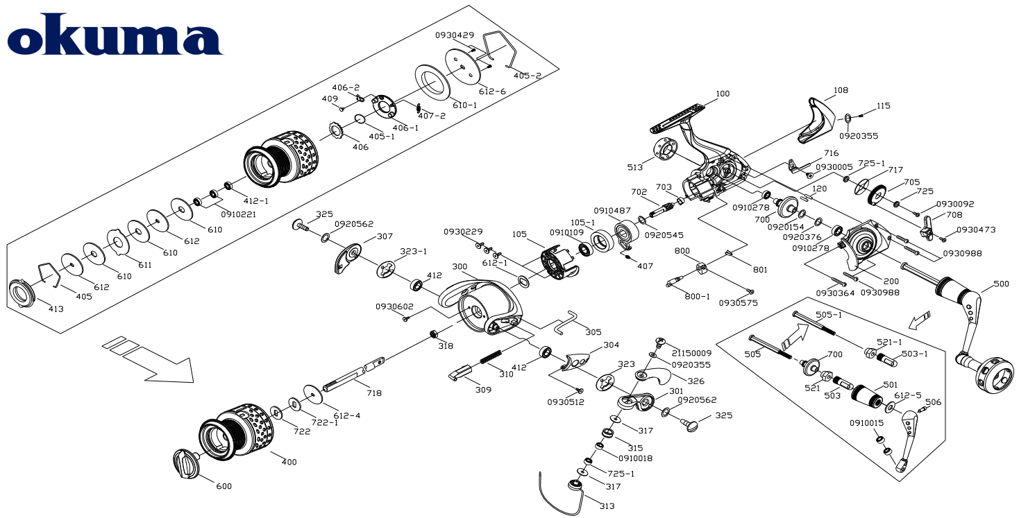
SA II-5000a 零件清單
