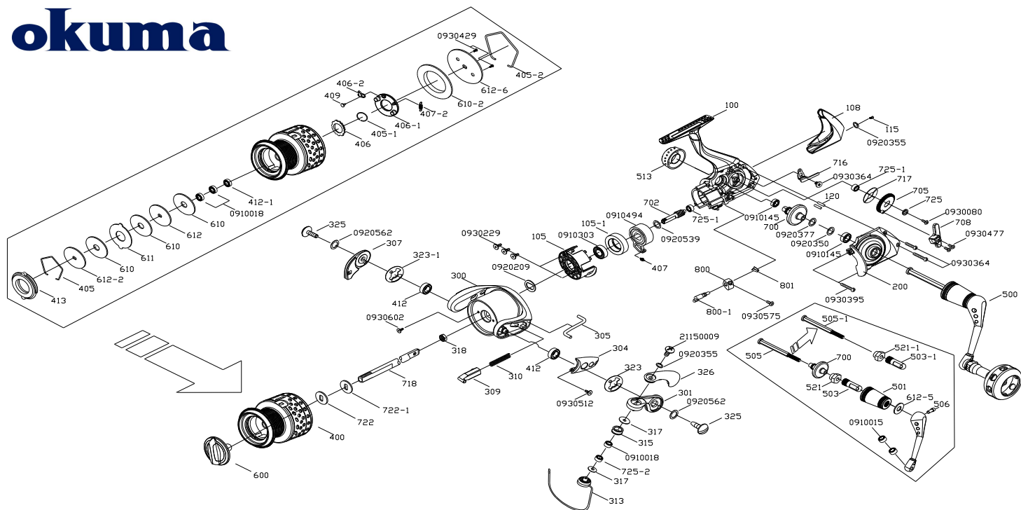
SA II-10000a 零件清單
