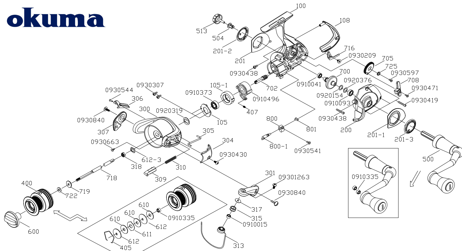
Pisces II-2000 零件清單
