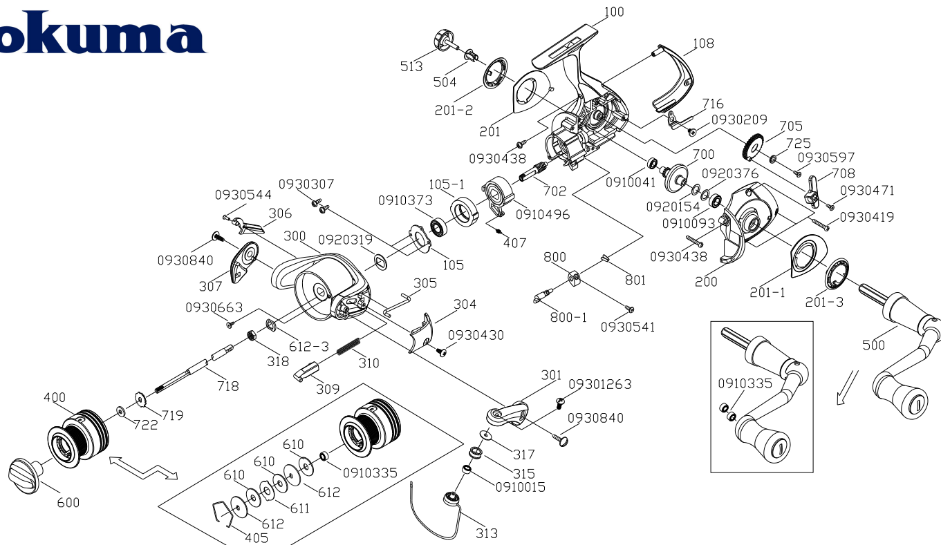
Pisces II-2000M 零件清單
