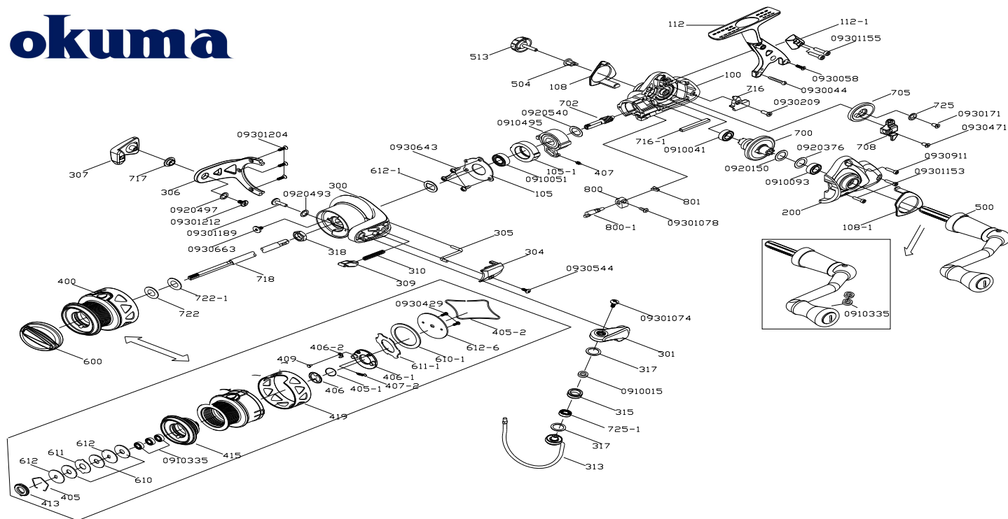
Trio-30 零件清單
