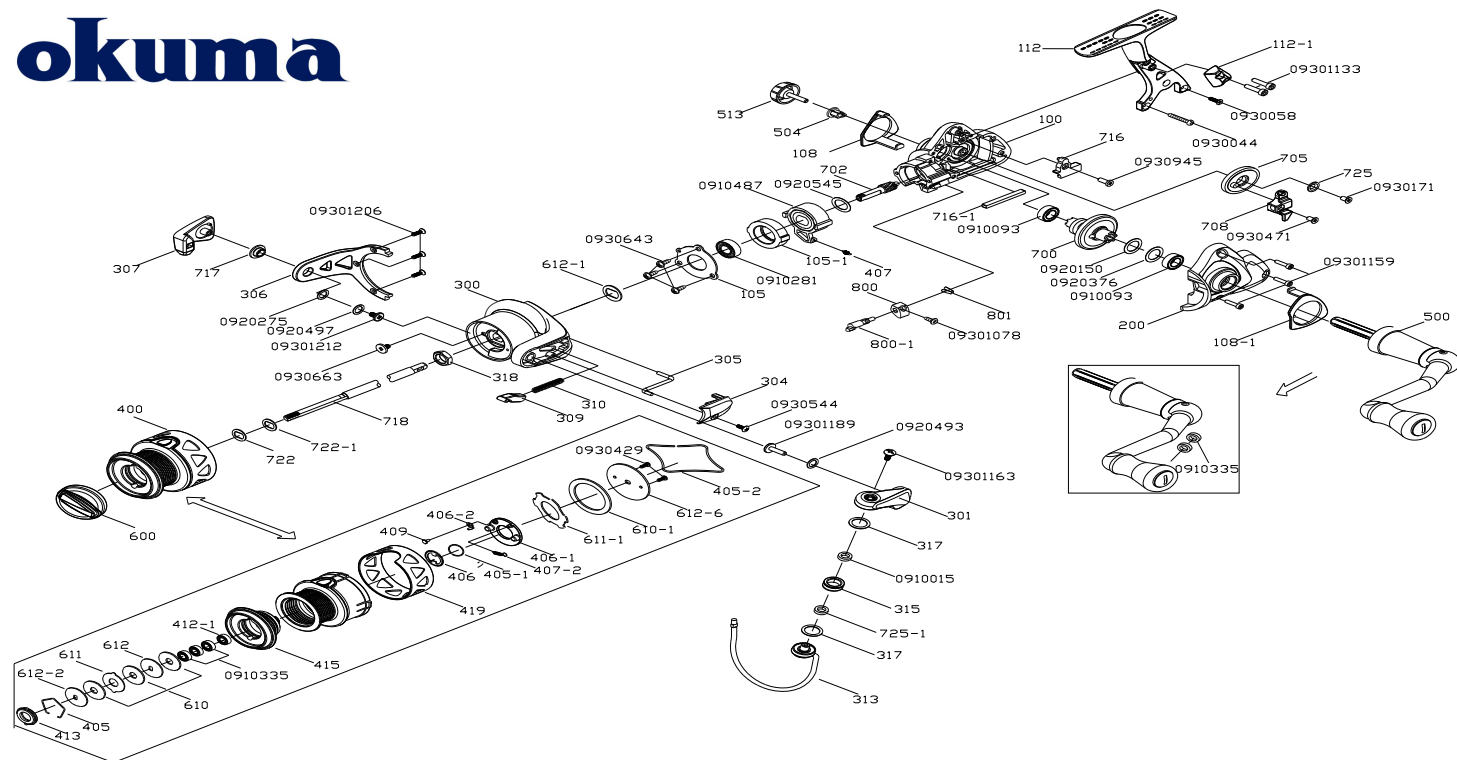
Trio-55 零件清單
