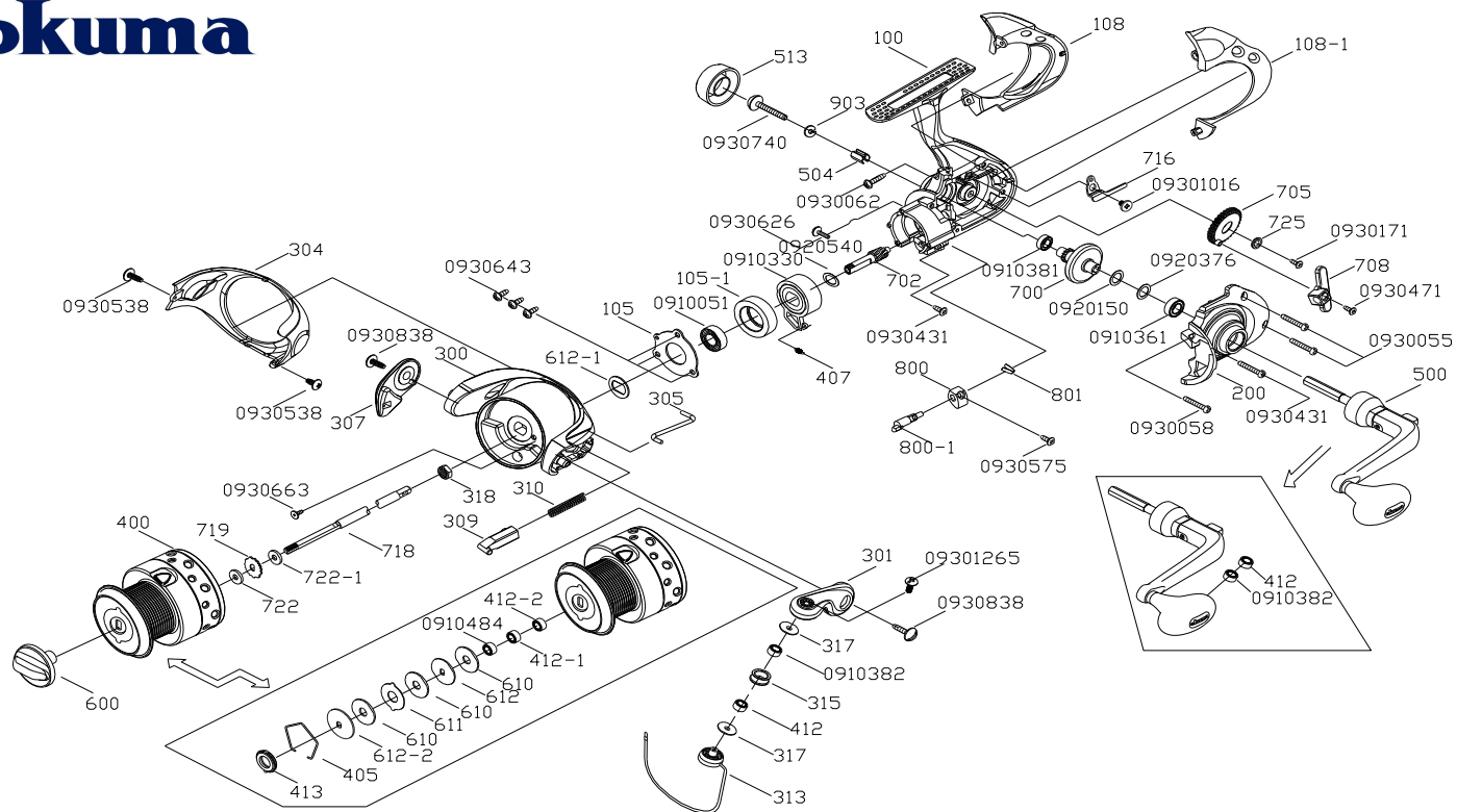
LOE-3000 零件清單
