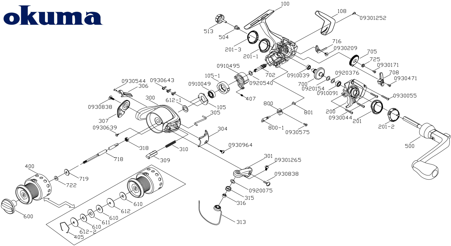
SPa-4000 零件清單
