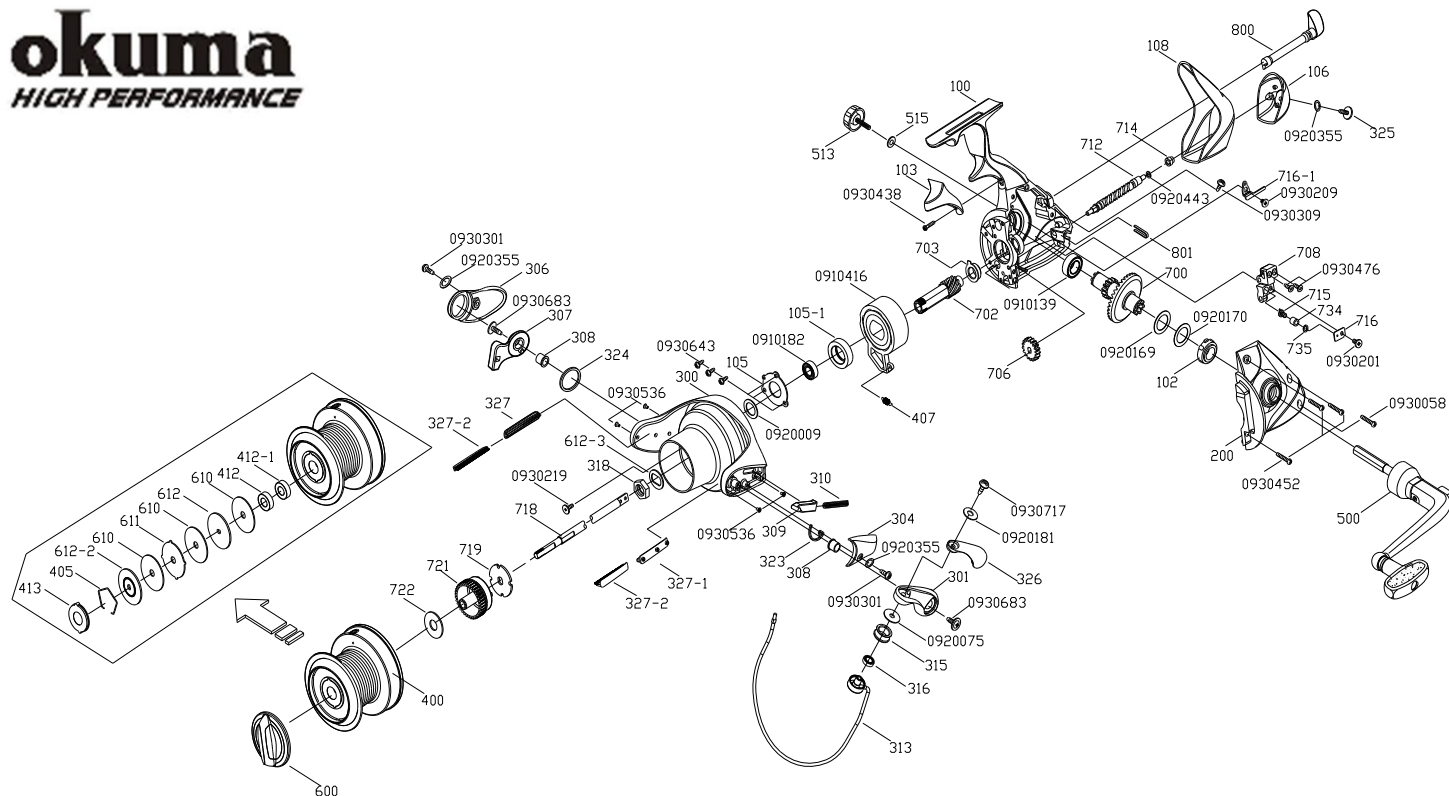
LR-10000 零件清單
