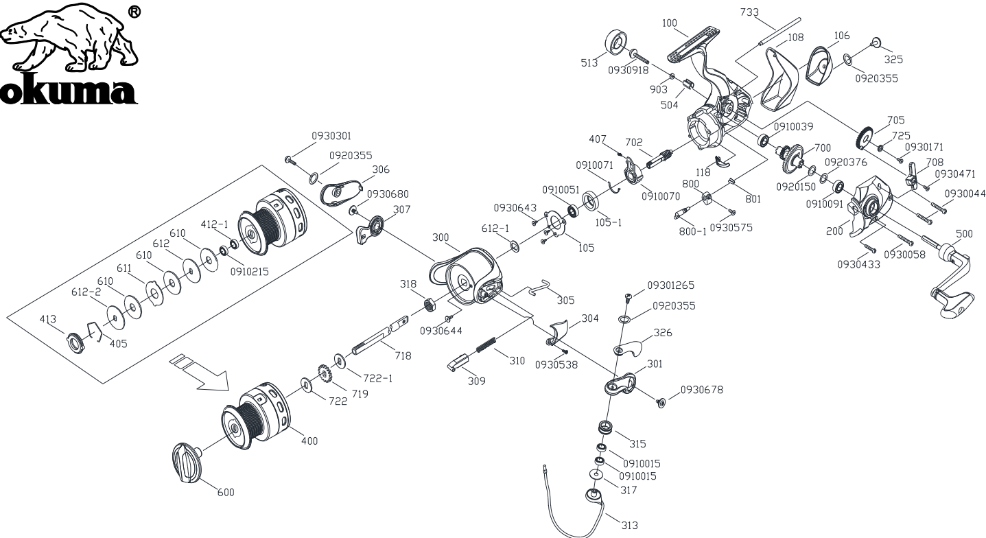
ET III-2000 零件清單
