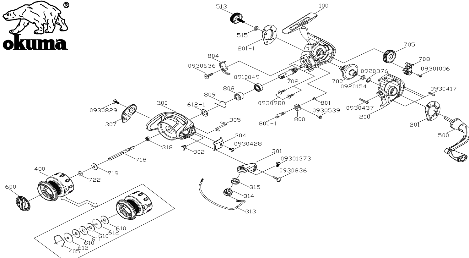
CA-30 零件清單
