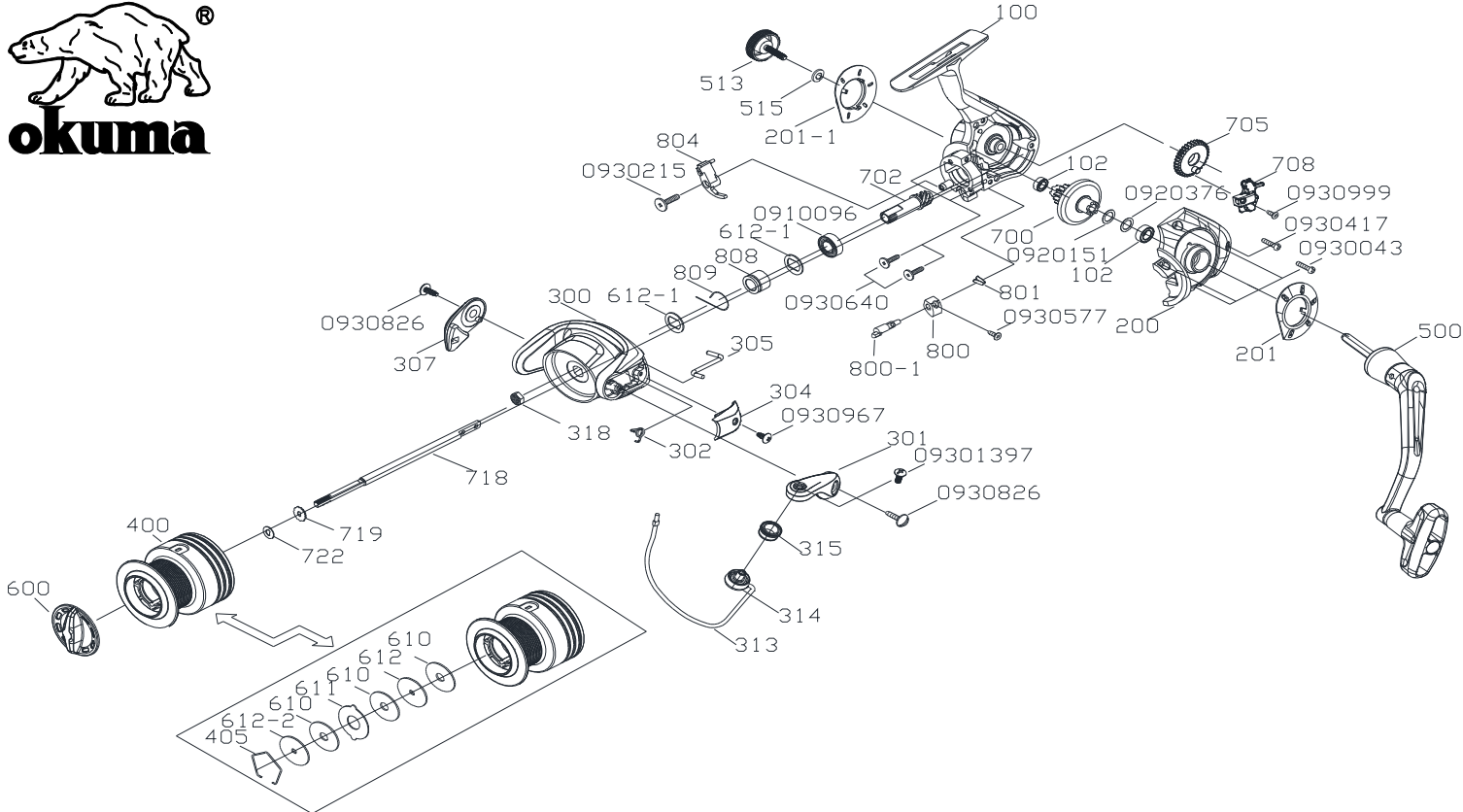
Nx-55 零件清單
