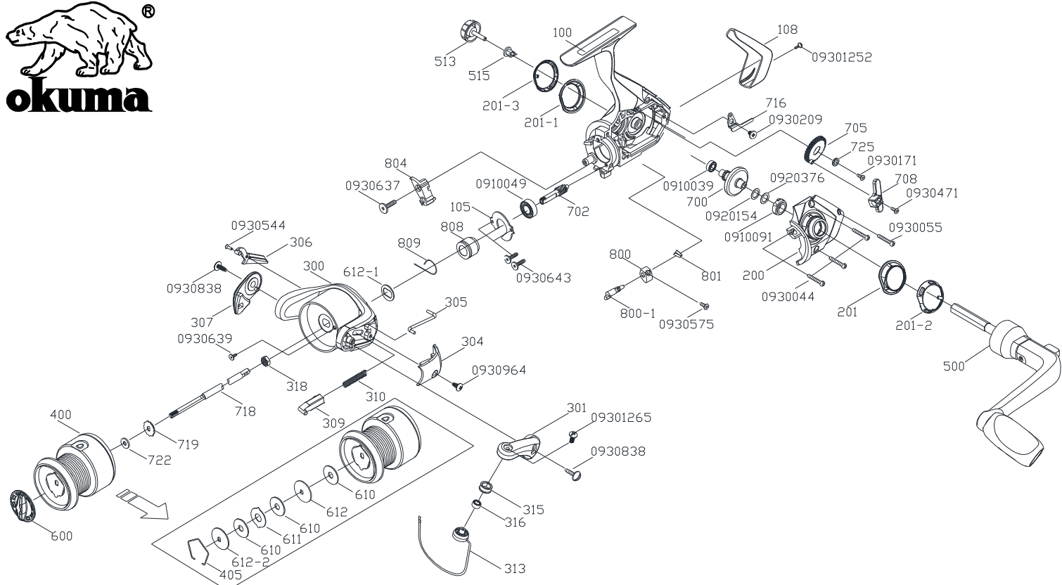
SNa-4000b 零件清單
