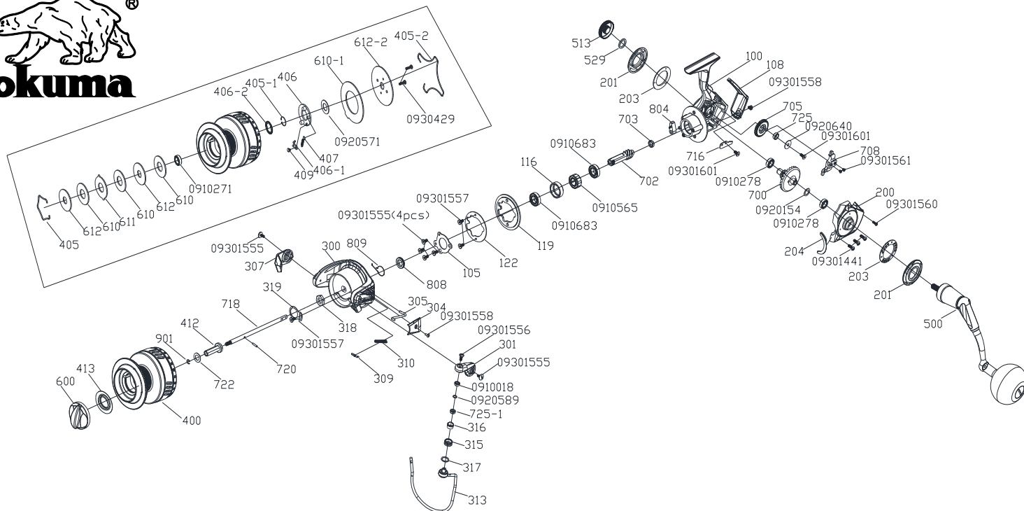
CJ-14000 零件清單
