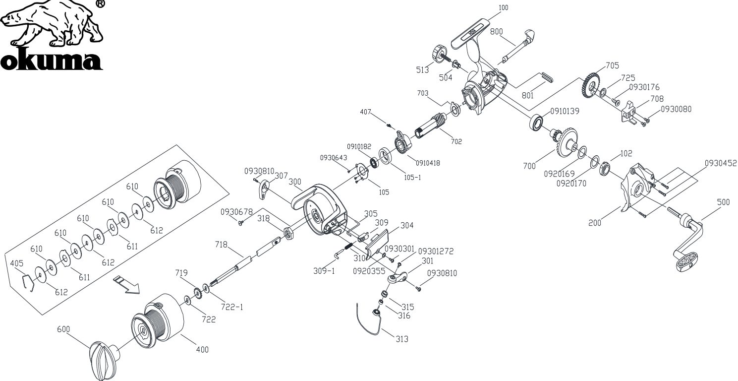
LBIII-6000 零件清單
