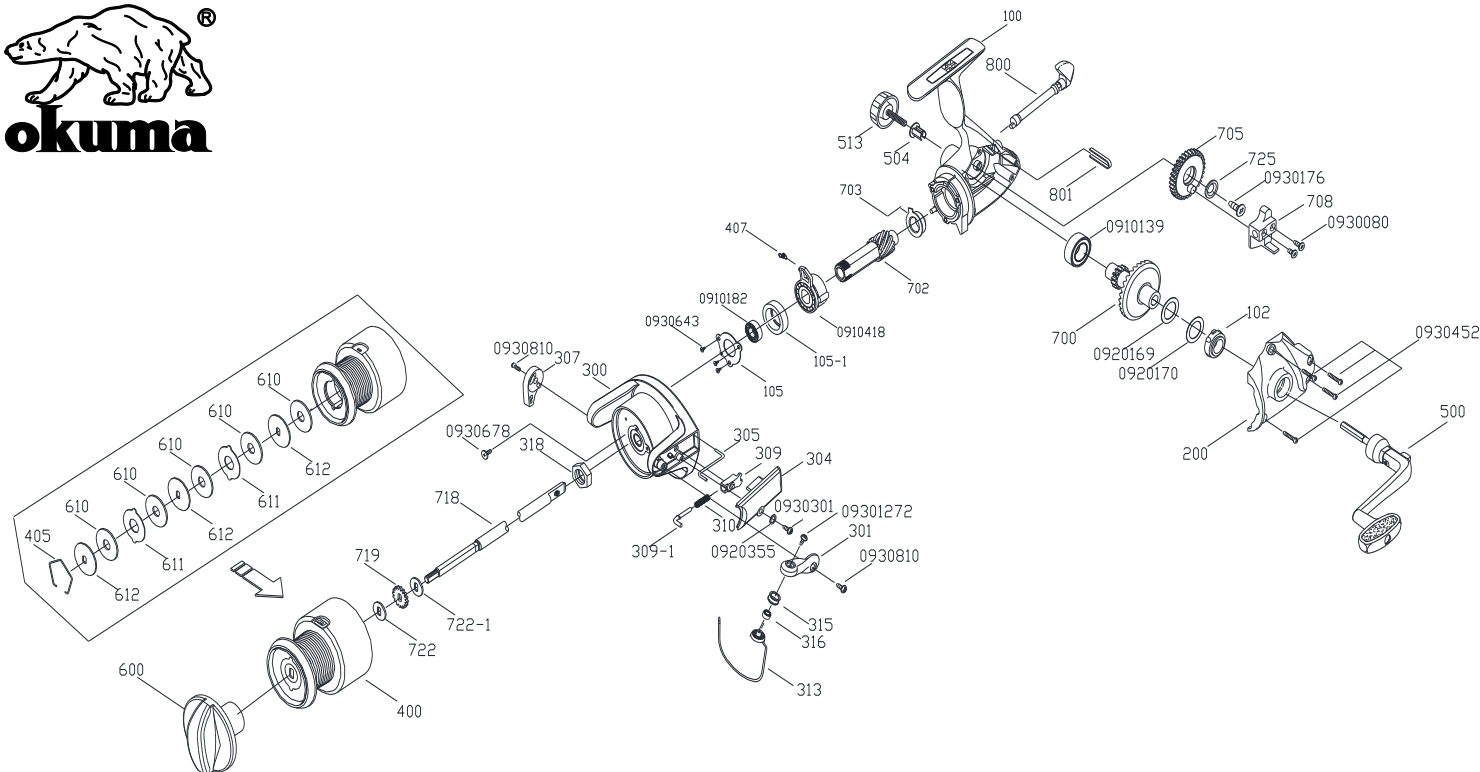
LBIII-7000 零件清單
