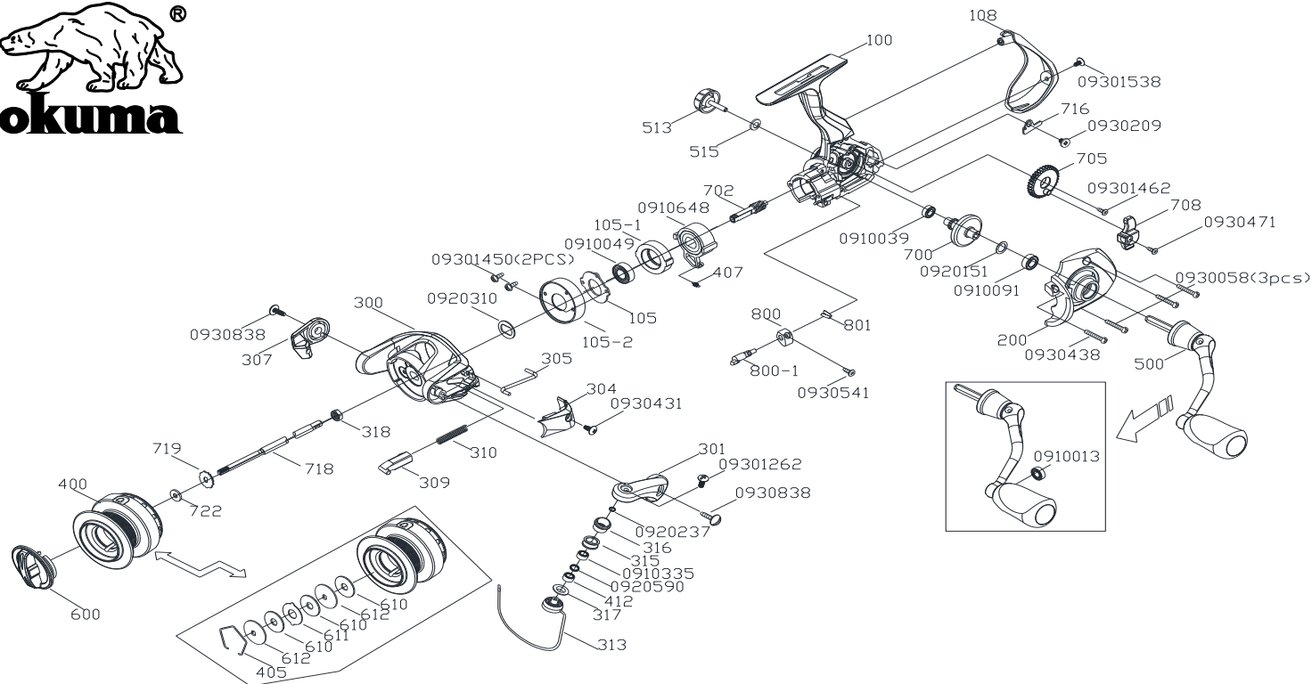
NMS-C4000 零件清單
