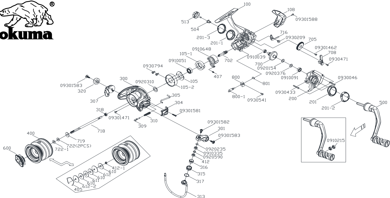
PS III-2000 零件清單
