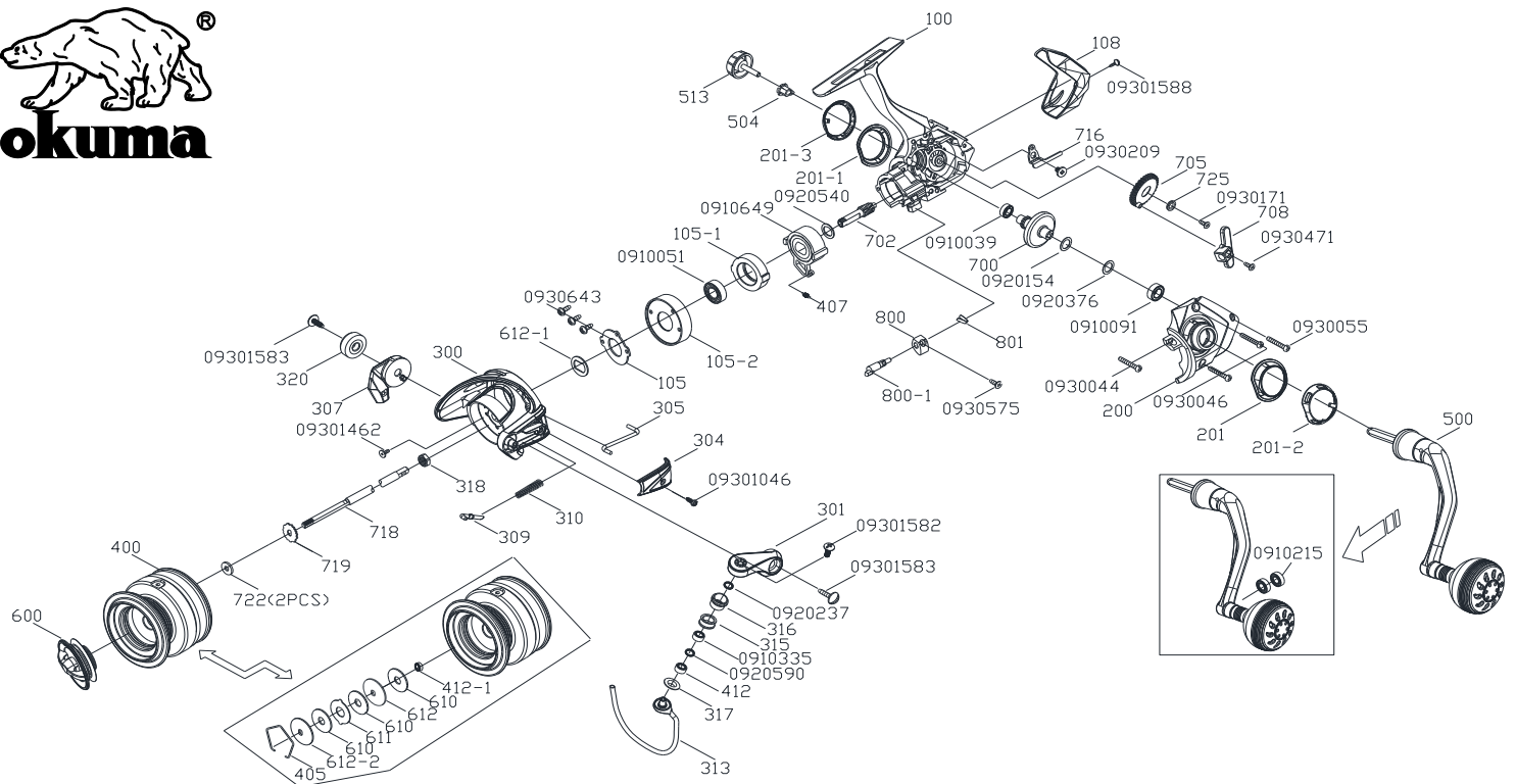
PS III-4000 零件清單
