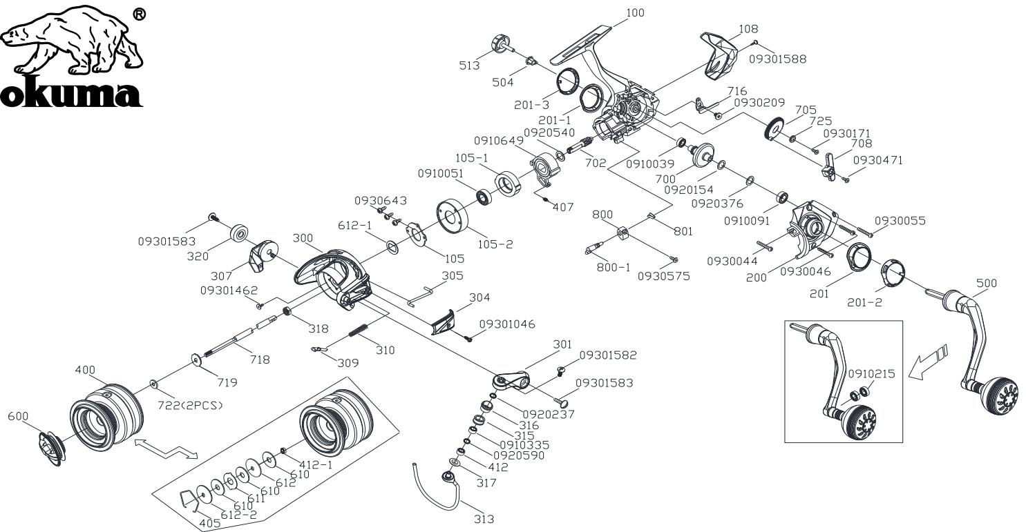
PS III-5000 零件清單
