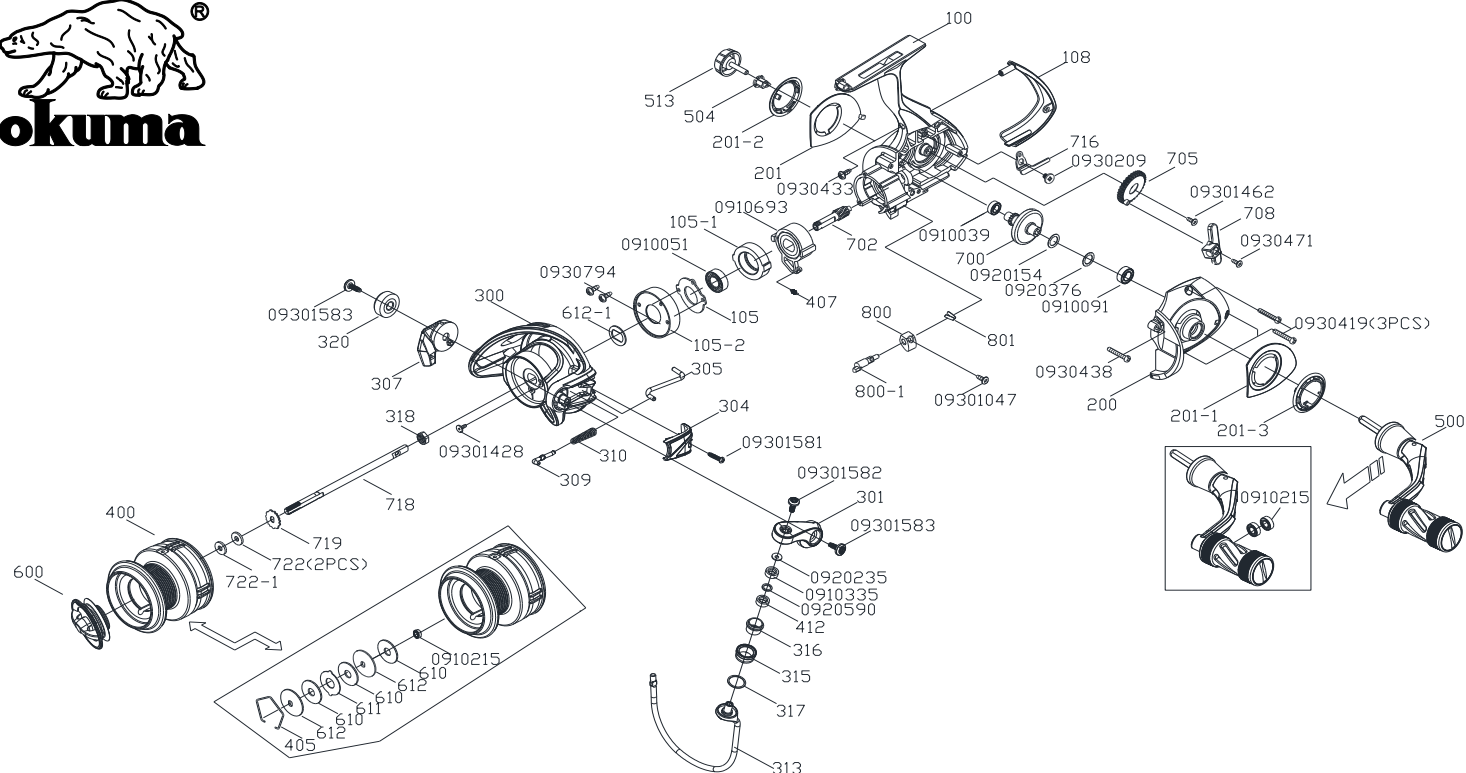
RTX II-3000 零件清單
