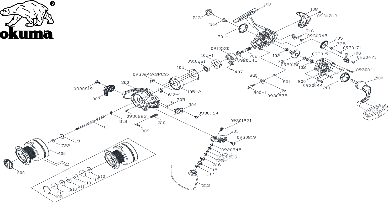
SN-6000 零件清單
