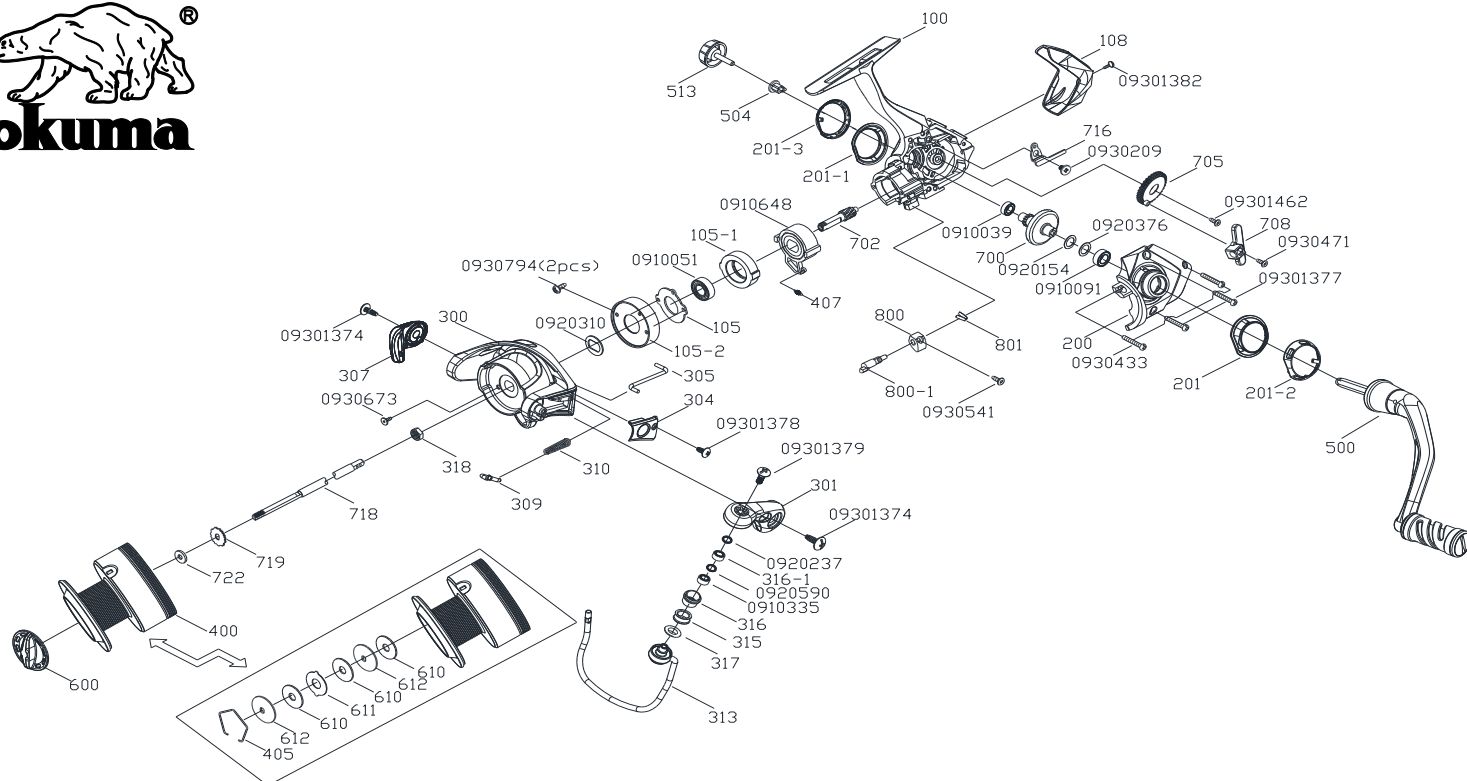
SPa II-2500 零件清單
