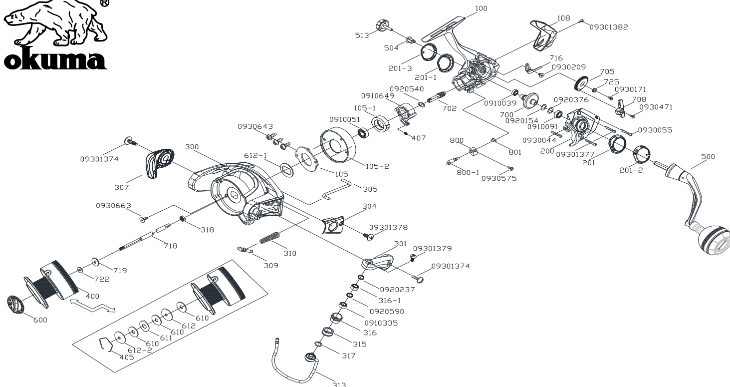
SPa II-5000 零件清單
