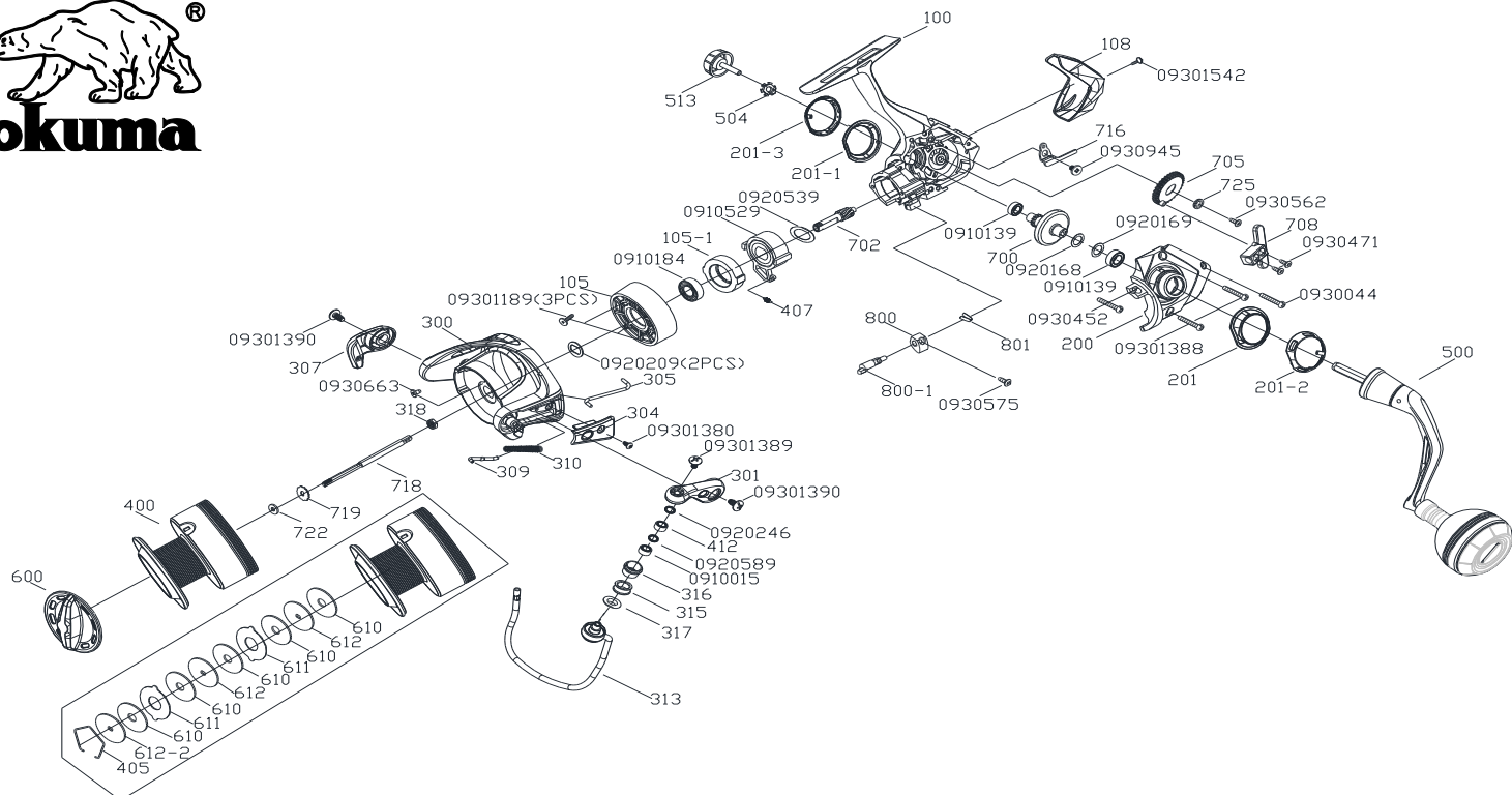
SPa II-14000 零件清单
