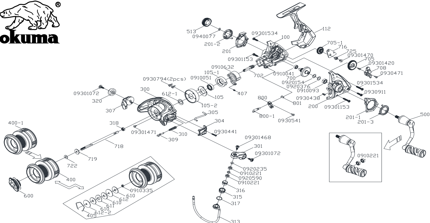
Epixor TW-3000 零件清單
