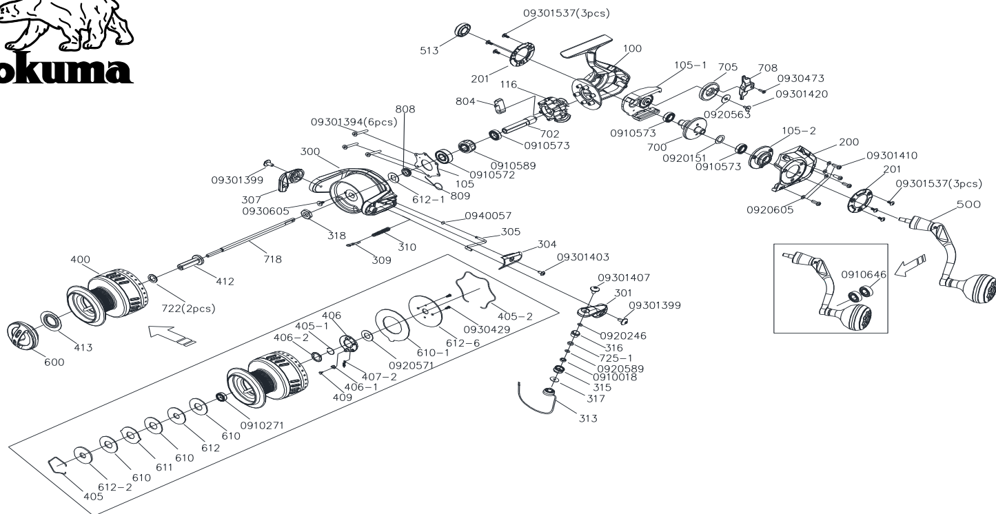
AZORES-8000P 零件清單
