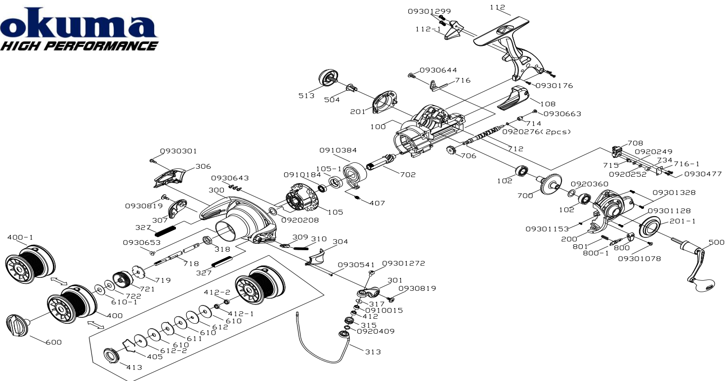
TS-6000 零件清單
