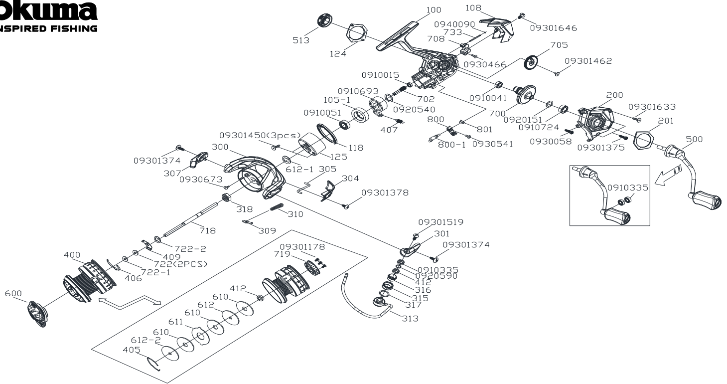
CHD-2500A 零件清單
