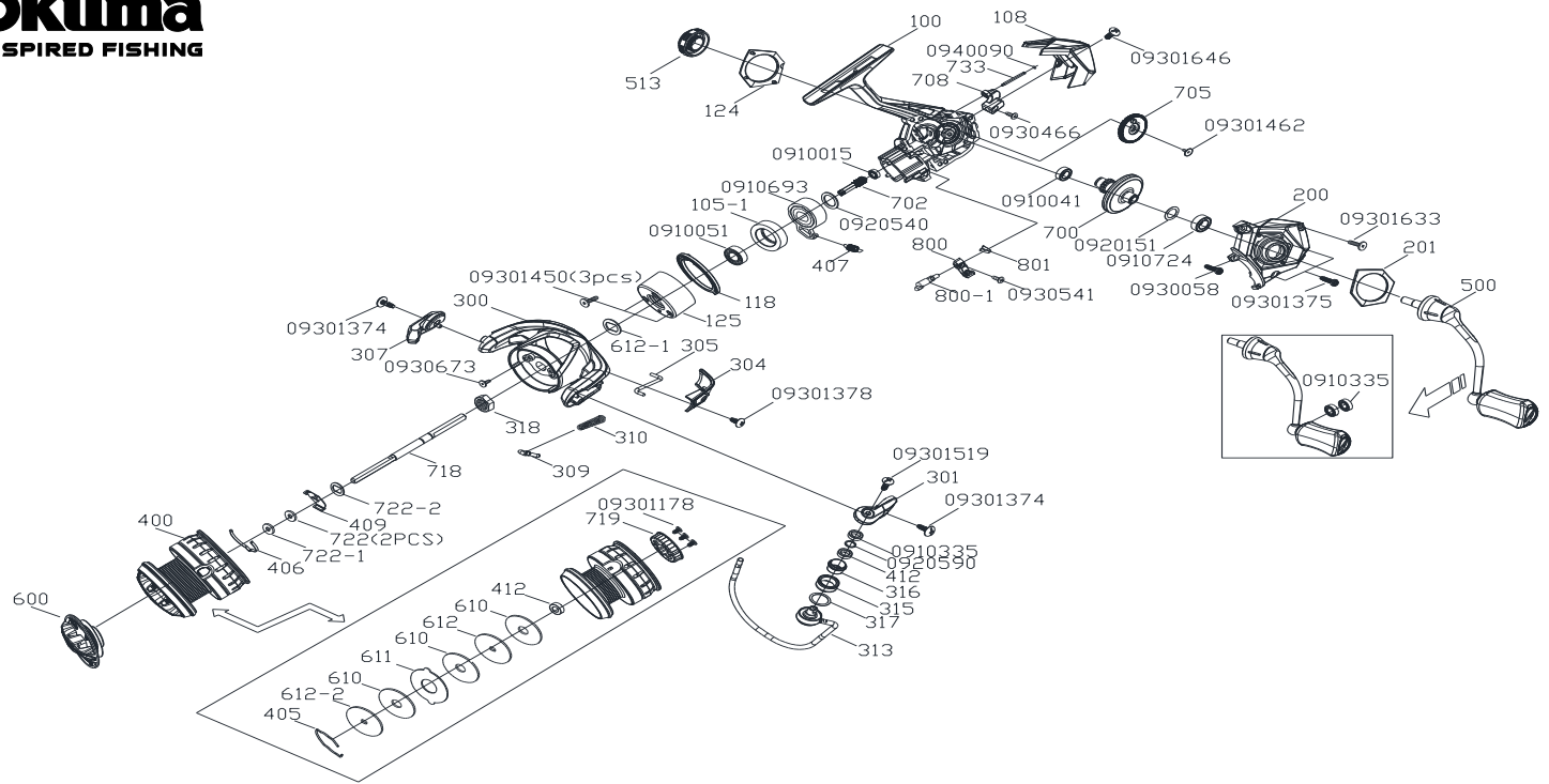
CHD-2500SA 零件清單
