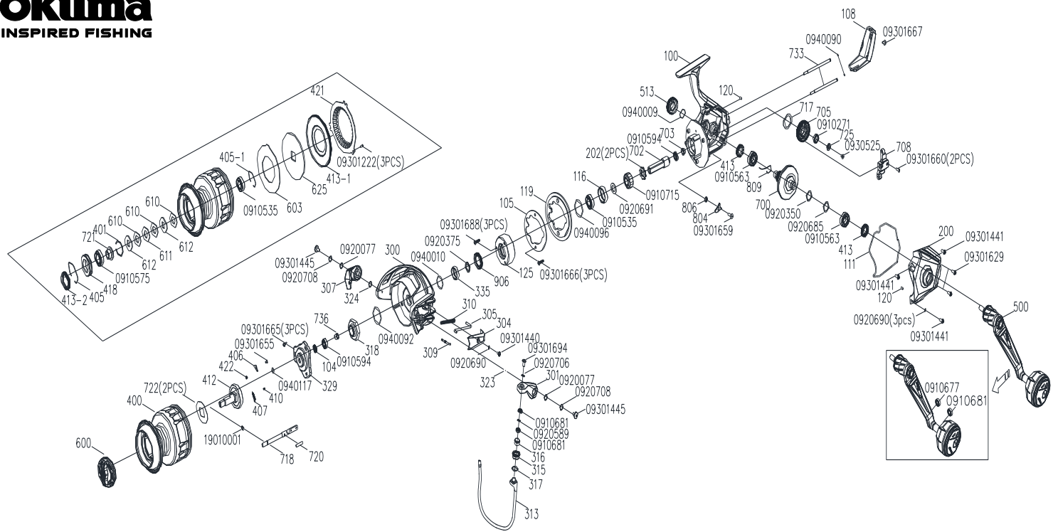
TSR-10000PA 零件清單
