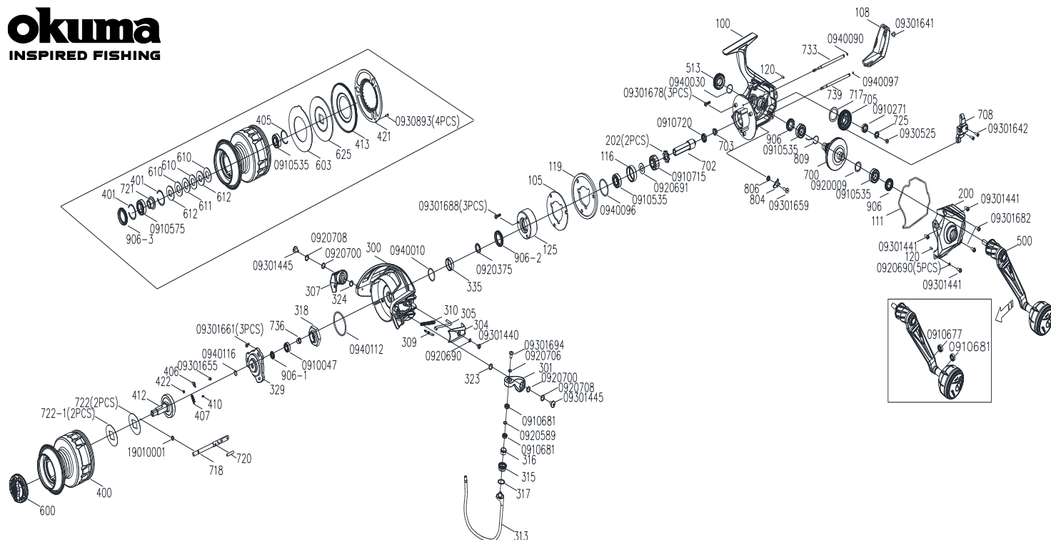
TSR-20000PA 零件清單
