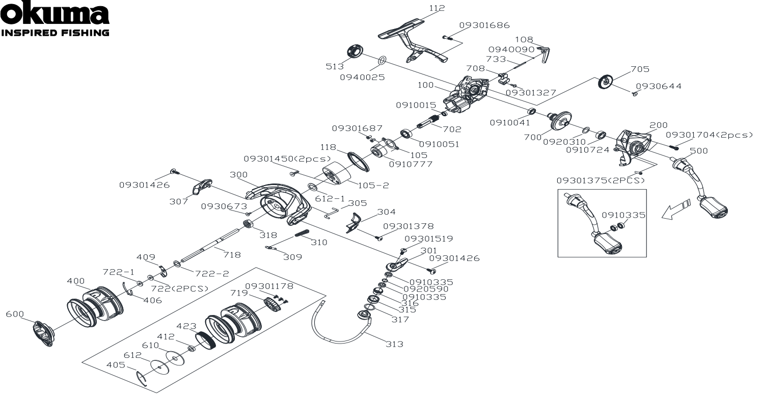
ISX-C2000HA 零件清單
