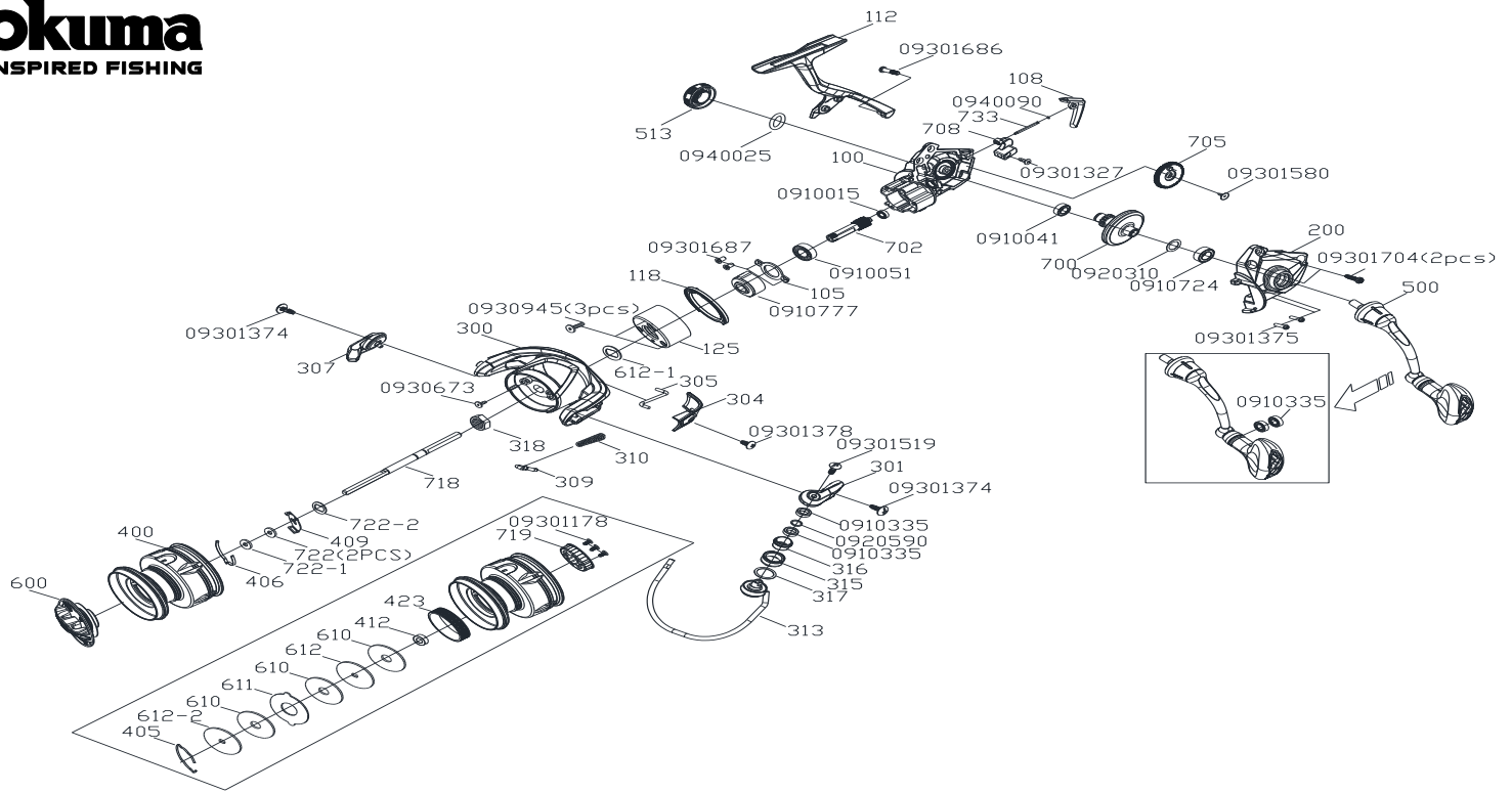
ISX-C5000XA 零件清單
