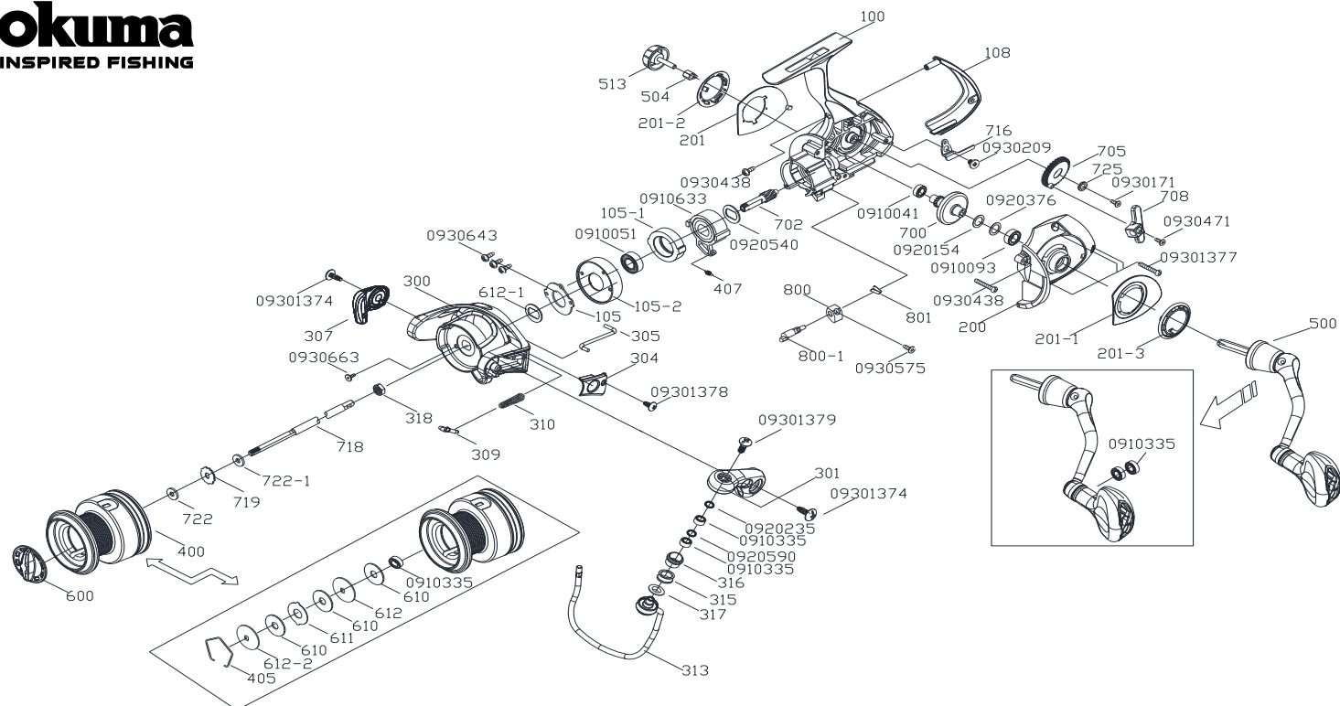
SD-C5000 零件清單
