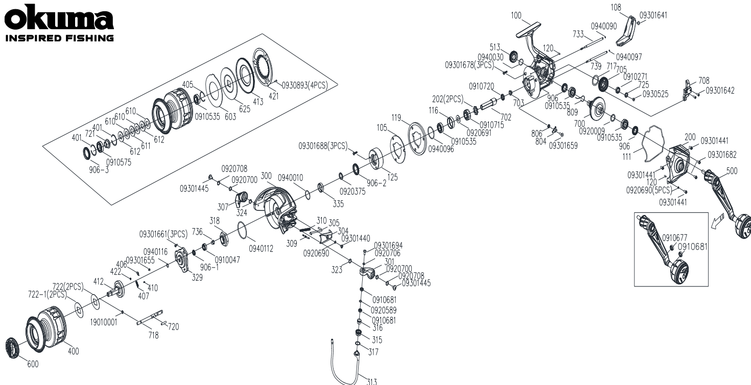
TSR-18000PA 零件清單
