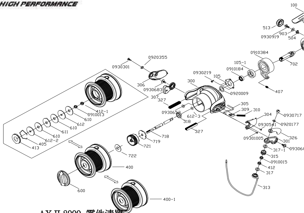
AX II-8000 零件清單
