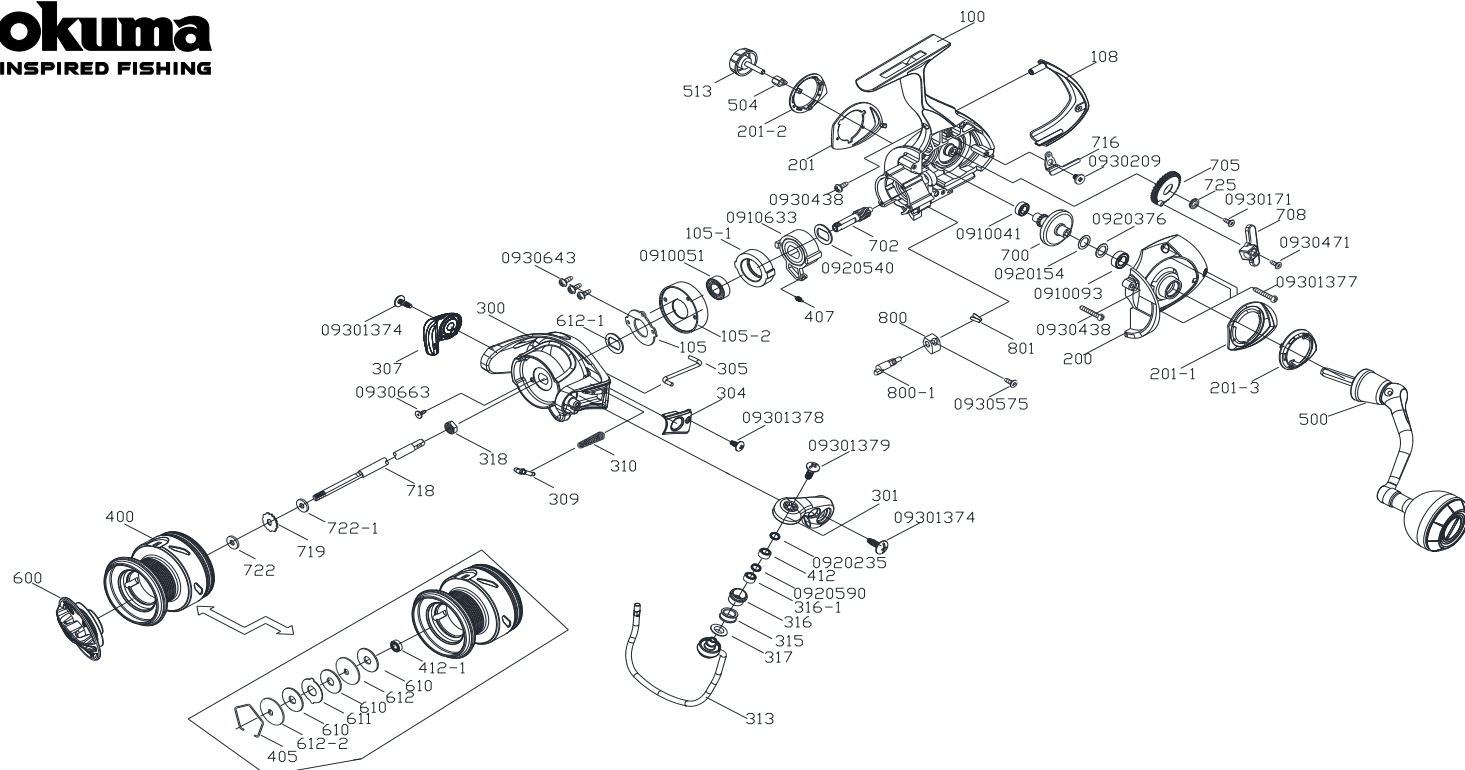
PS-4000A 零件清單
