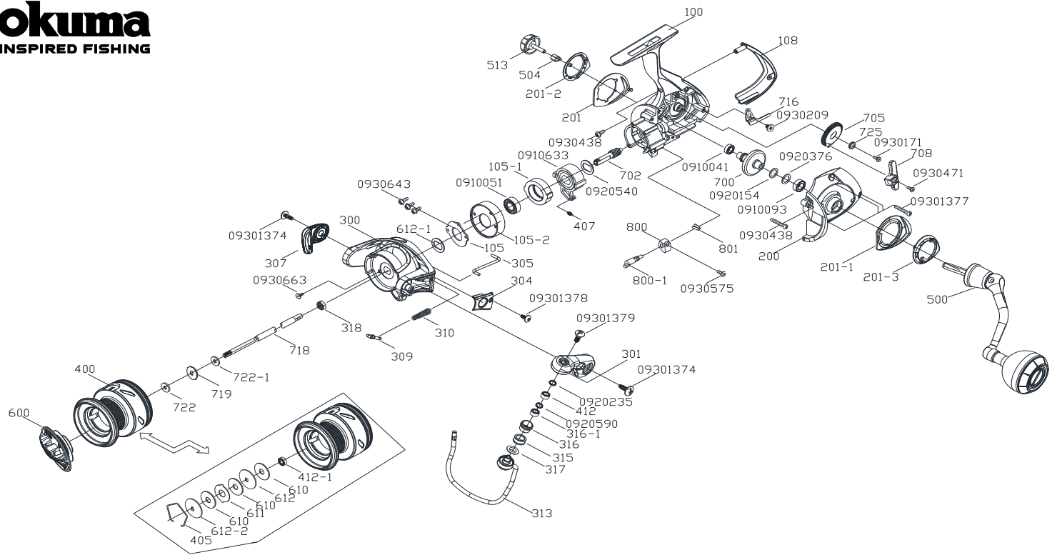
PS-C5000A 零件清單
