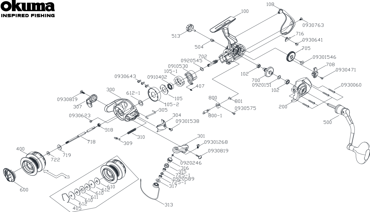
WPR-6000A 零件清單
