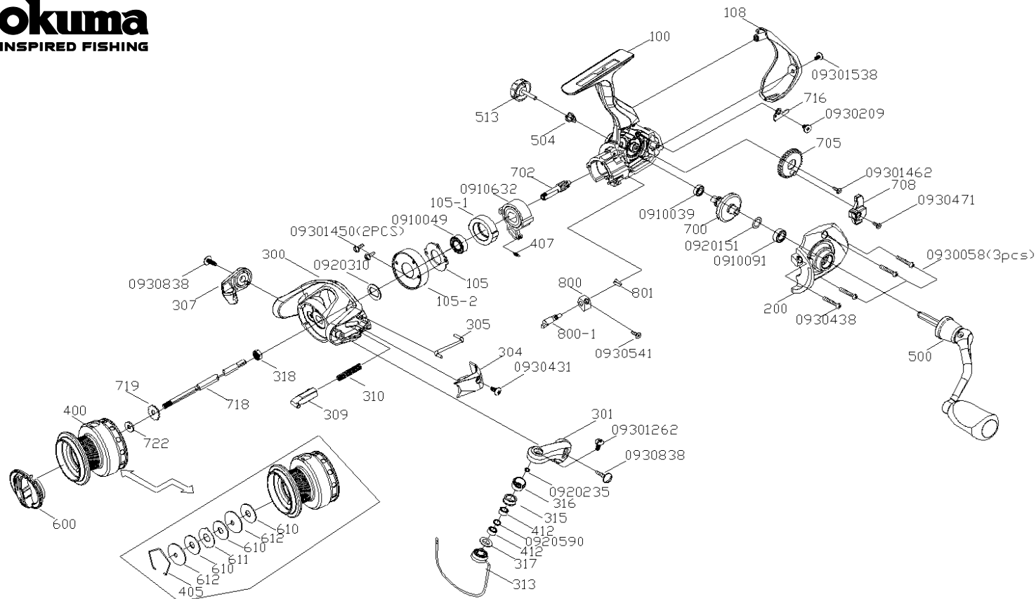
WPR-2000A1 零件清單
