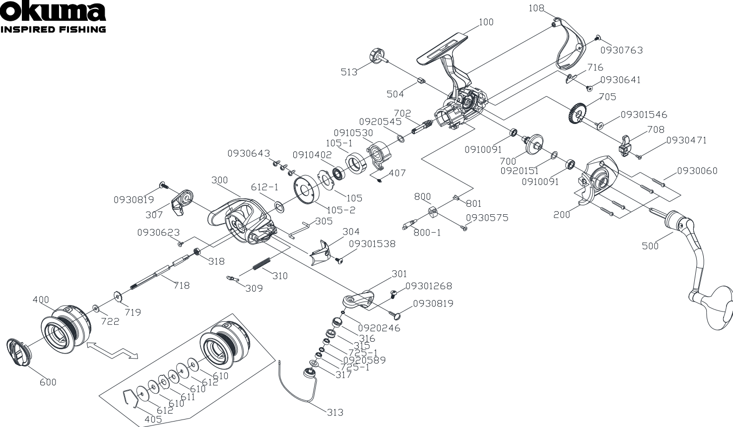
WPR-6000A1 零件清單
