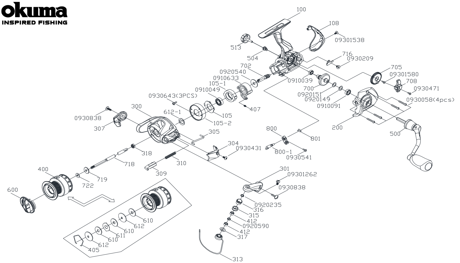
WPR-4000A1 零件清單
